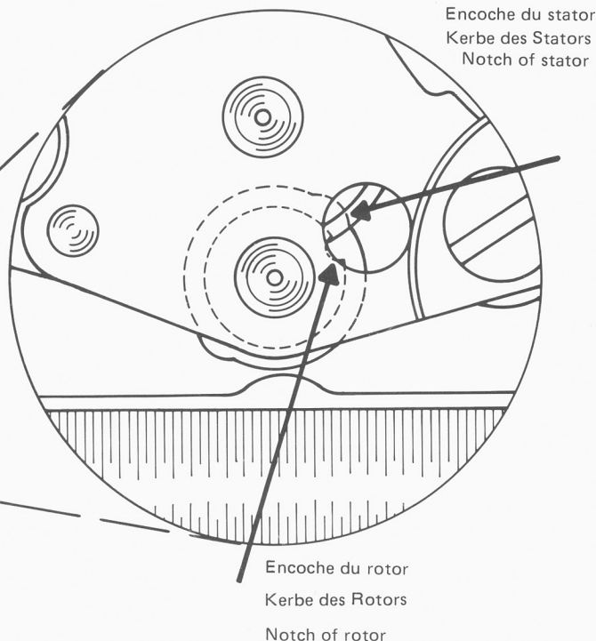
Encoche du rotor Kerbe des Rotors Notch of rotor
